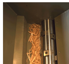
Rotor/knife Rotor/kniv
